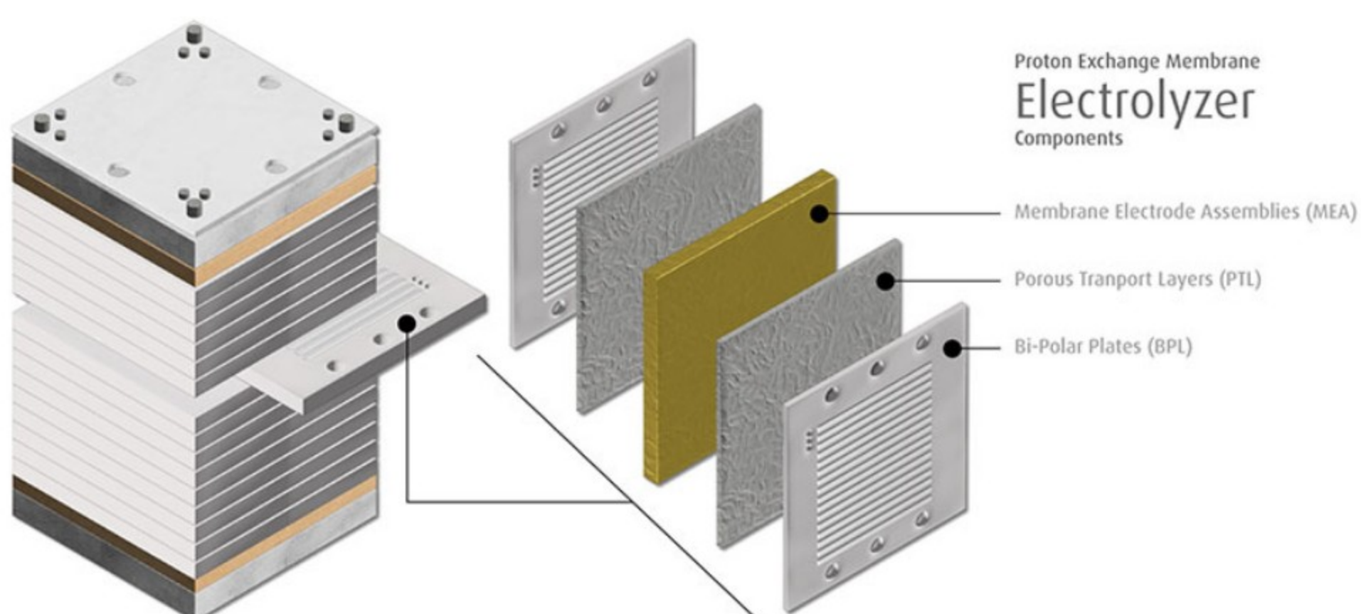
Bipolarplatten (Bipolar Plate, BPL) und poröse Transportschichten (Porous Transport Layers, PTL) aus platinierter Titan macht die Protonenaustauschmembran-Elektrolyse (PEM) deutlich leistungsfähiger. (Bild: Umicore)
