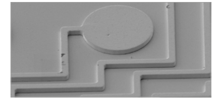
鍍金線條與凸點
