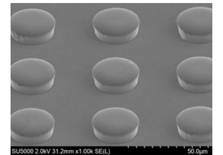
凸點鍍有 NiRUNA ® SC (不含硼酸的電解液)
