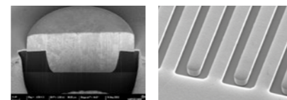
微孔測試 直徑 30 μm·深度 20 μm RDL (再佈線層) 2um/2um 線寬/線距
