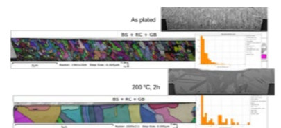
上圖: 細晶粒銅層 (晶粒 < 100 nm); 底部: 退火後晶粒成長因子 > 5
