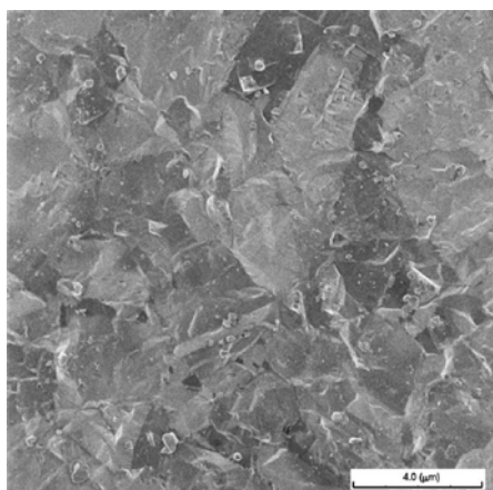
REM-Oberflächenbild eines DIG-Überzugs
