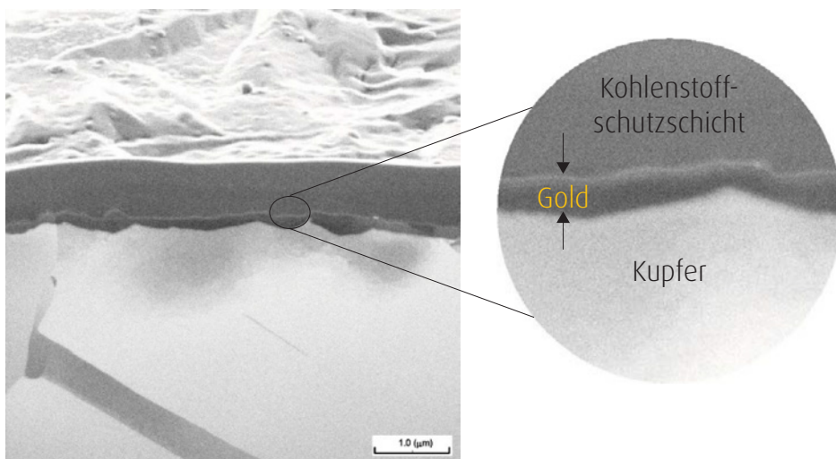
Querschnittsaufnahme eines DIG-Überzugs mit FIB
